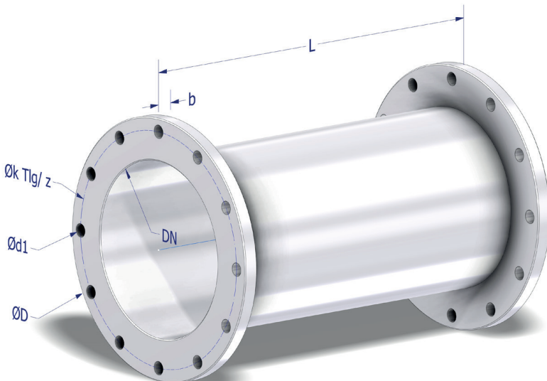
■ FFS-Stück; auch mit Mauerkragen lieferbar / FFS-fitting; also available with wall collar
