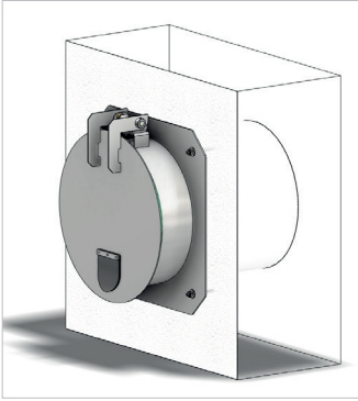
■ GW-RDD_DN: Rückstauklappe mit Entlastungs- klappe zum Andübeln / GW-RDD_DN: discharge flap for dowel-mounting
