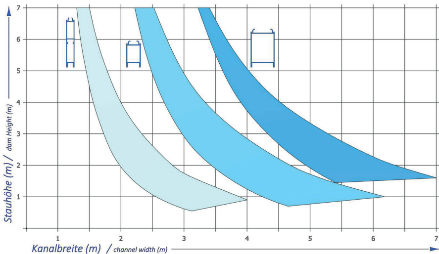
■ Dammbalken-Auswahltable / stop log selection table
