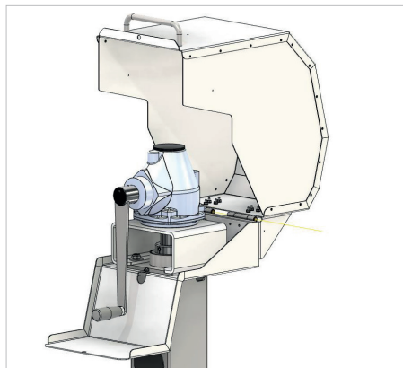
▪ Abdeckhaube für Getriebe mit Handkurbel / cover for gearbox with crank handle
