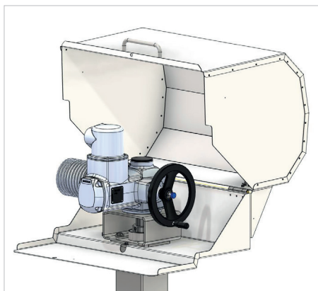
▪ Abdeckhaube für E-Antrieb / cover for electric drive
