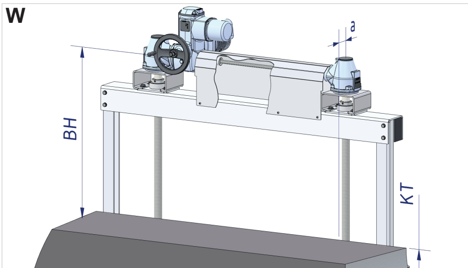
▪ Antrieb 2-spindelrig auf Traverse mittels Kegelradgetrieben und E-Antrieb / 2-spindle drive mounted on crossbar with bevel gearboxes and electric actuator
