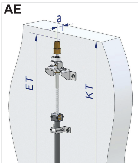
▪ Antrieb im Schacht mittels Vierkant und Stellungsanzeige / drive mounted in chamber with square-head and position indicator
