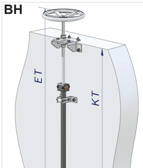
▪ Antrieb auf Mauerkrone mittels Handrad / drive mounted on wall plate with hand wheel
