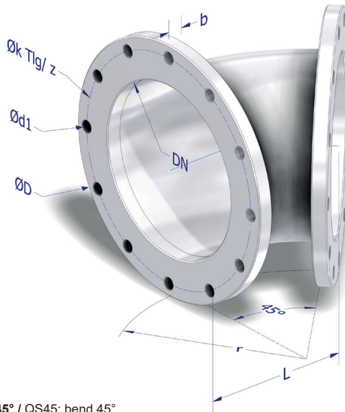
■ QS45: Rohrbogen 45° / QS45: bend 45°
