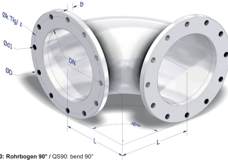
■ QS90: Rohrbogen 90° / QS90: bend 90°
