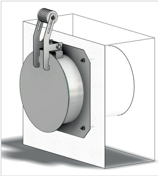
■ GW-RDD_HG: Rückstauklappe mit Hebel und Gegengewicht / GW-RDD_HG: flap valve with lever and counterweight
