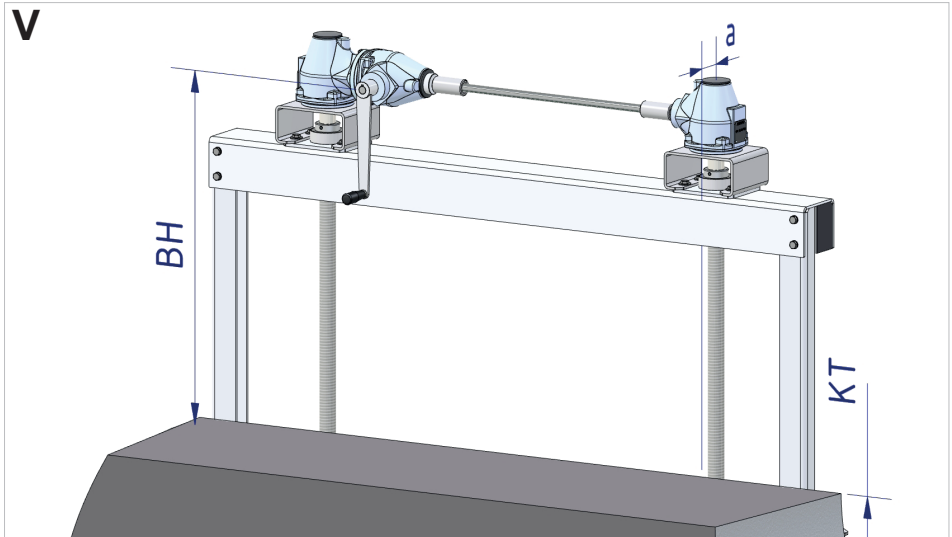
▪ Antrieb 2-spindelrig auf Traverse mittels Kegelradgetrieben und Handkurbel / 2-spindle drive mounted on crossbar with bevel gearbox and crank handle
