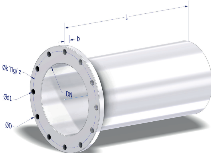
■ FS-Stück; auch mit Mauerkragen lieferbar / FS-fitting; also available with wall collar
