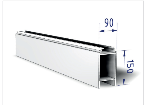
■ Typ B / type B: 7,22 kg/lfm
