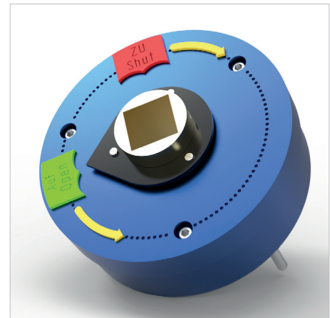
■ Wasserdichtes mechanisches Räderzeigerwerk aus Aluminium / waterproof mechanical position indicator made from aluminium
